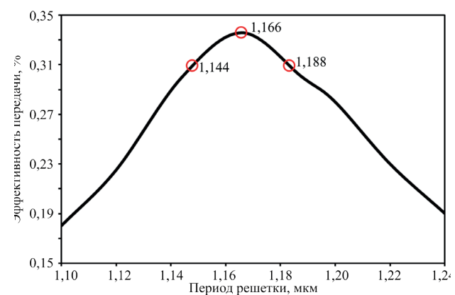
Рис. 6. Зависимость эффективности передачи от периода решетки
