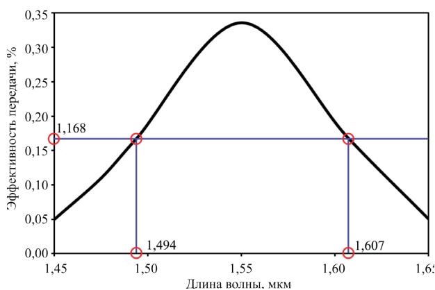
Рис. 5. Спектральная зависимость эффективности передачи ФРР после оптимизации
