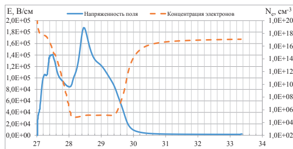
Рис. 2. Проекция напряженности электрического поля на направление тока и концентрация электронов вдоль границы раздела кремний / оксид кремния
